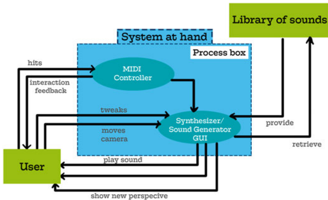
Level-1 DFD
